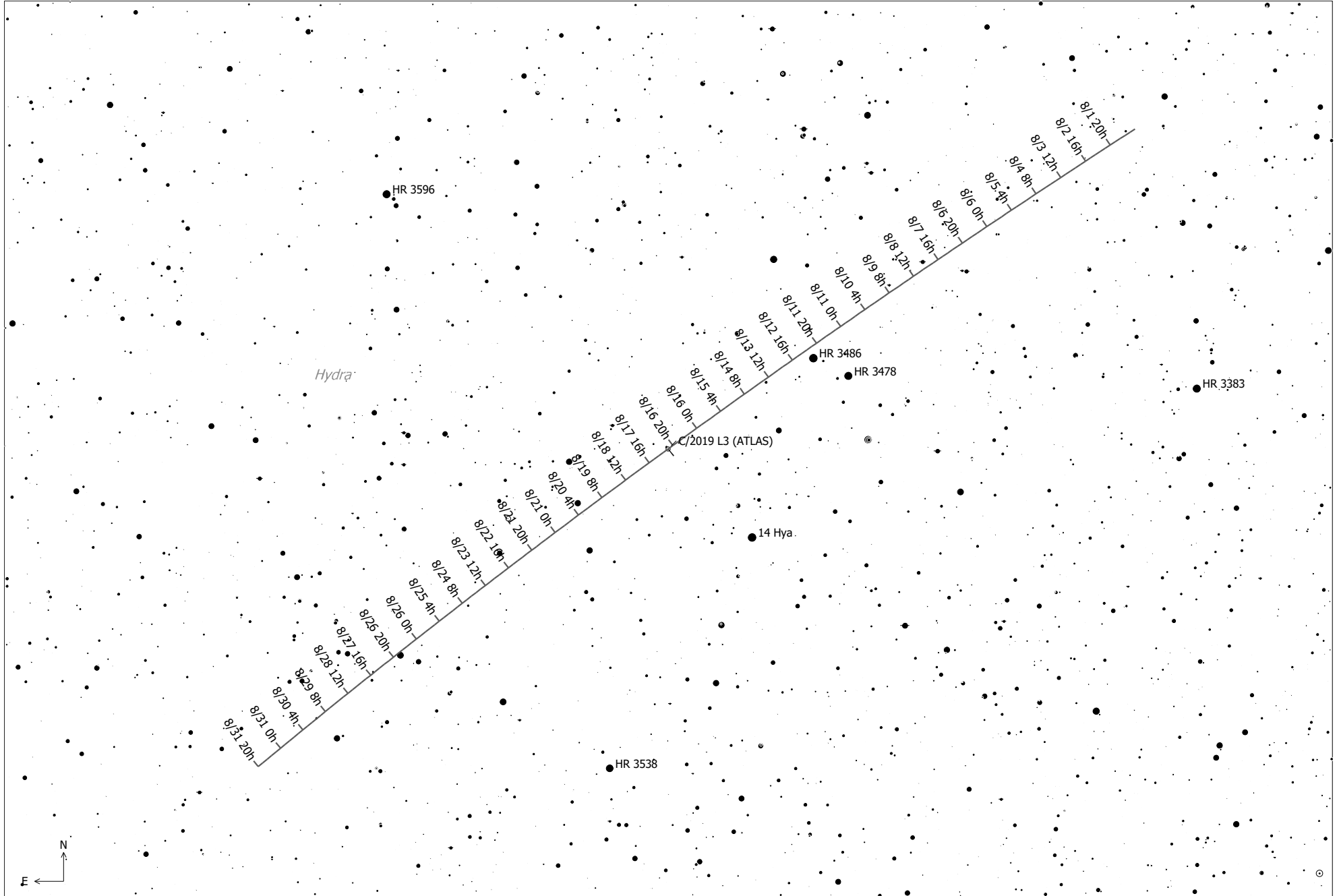
C/2019 L3 (ATLAS) (Comet)
