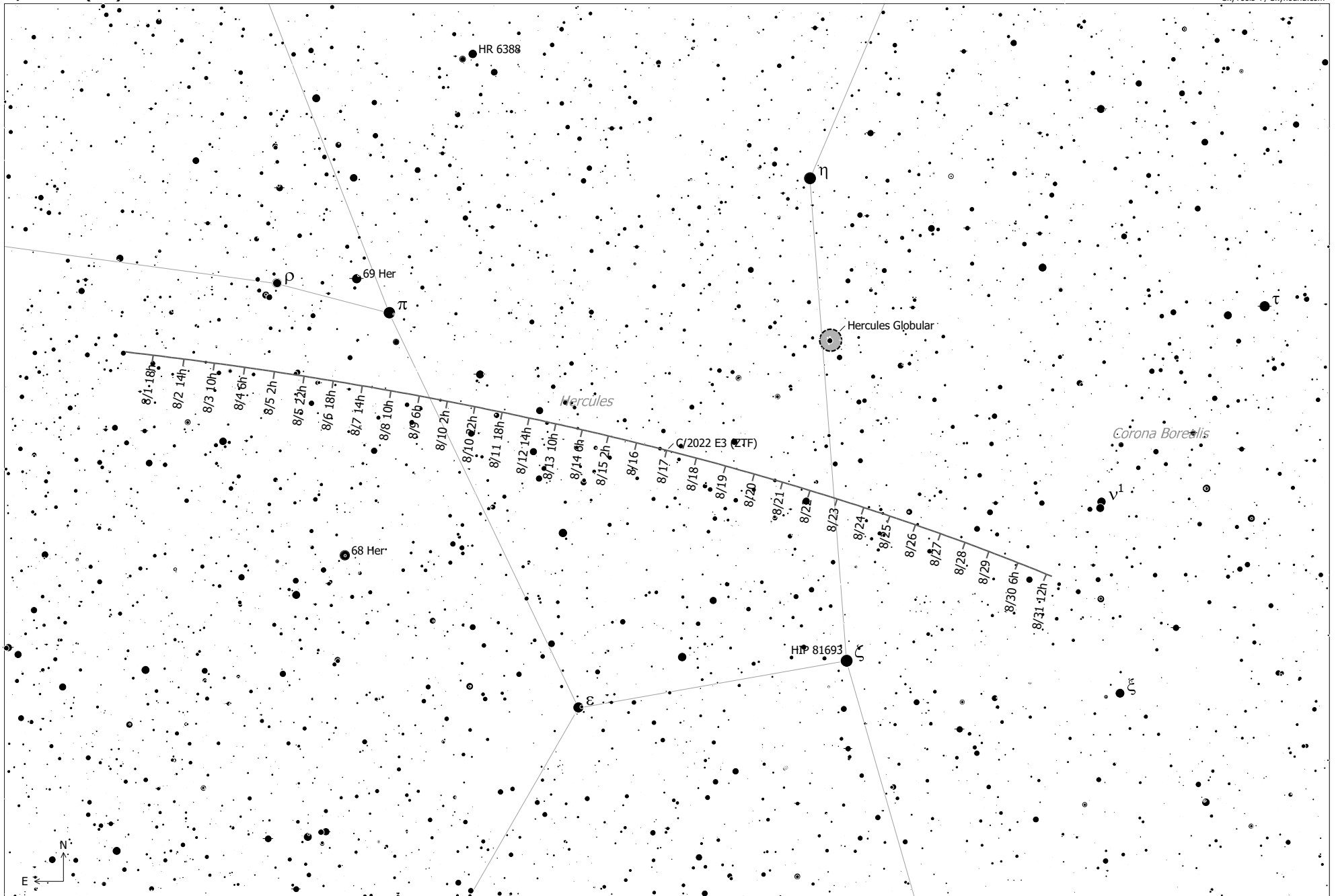
C/2022 E3 (ZTF) (Comet)
